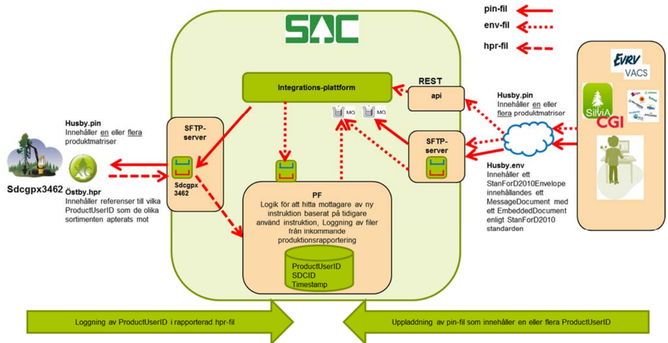
Figur 1 Översiktlig lösningsbeskrivning för produktionsstyrning
